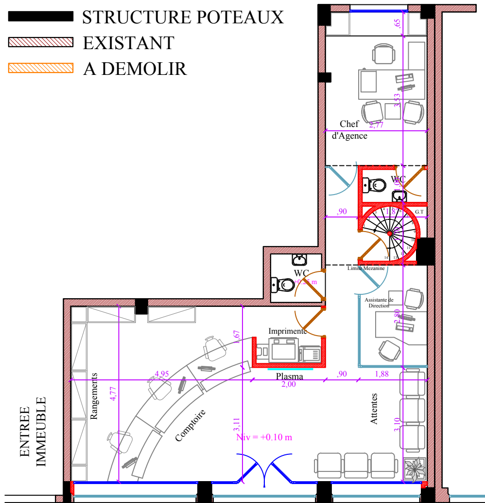
PLAN RDCH
