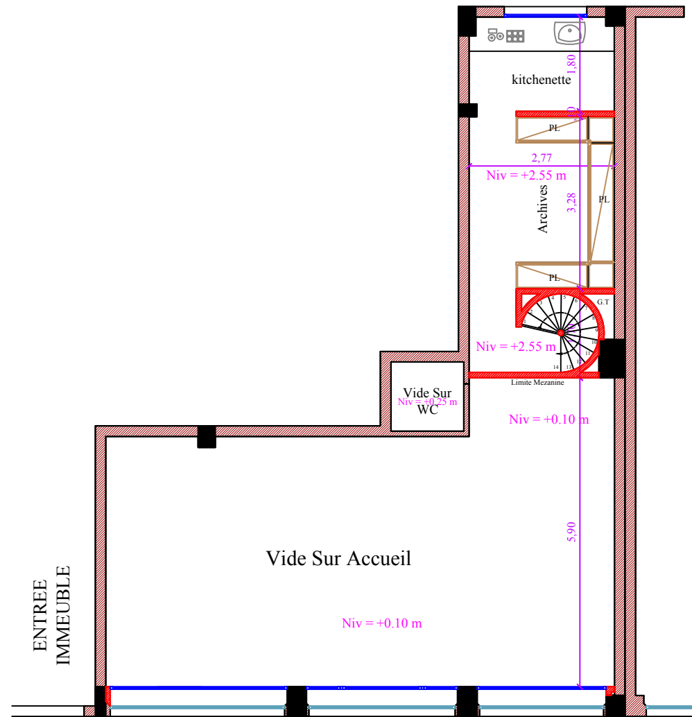
PLAN SOUPENTE
